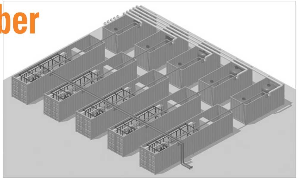
Esquema de la desalinizadora de cinco módulos.
